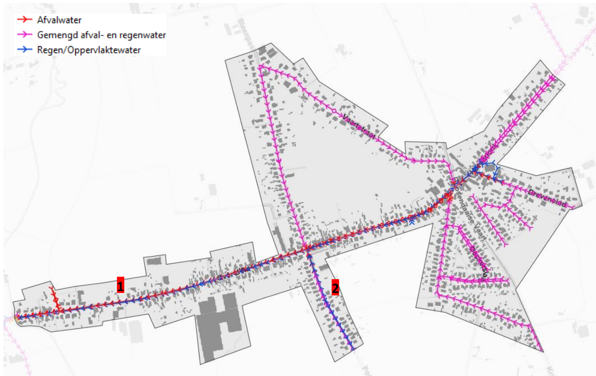
figuur 38. Huidige afwatering in woonkern Horendonk
