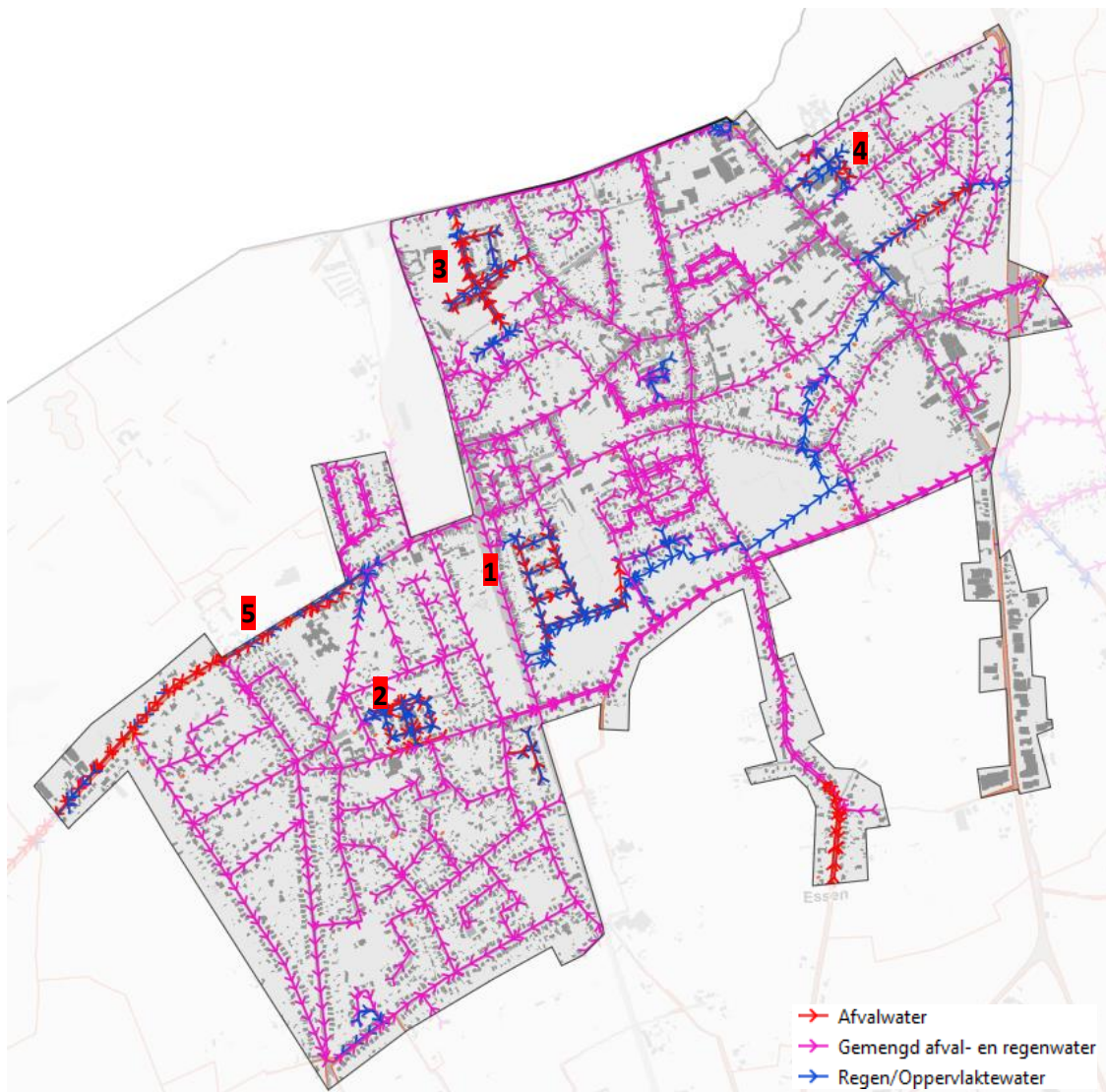
figuur 16. Huidige rioleringsysteem in woonkern Essen-Centrum en Heikant
